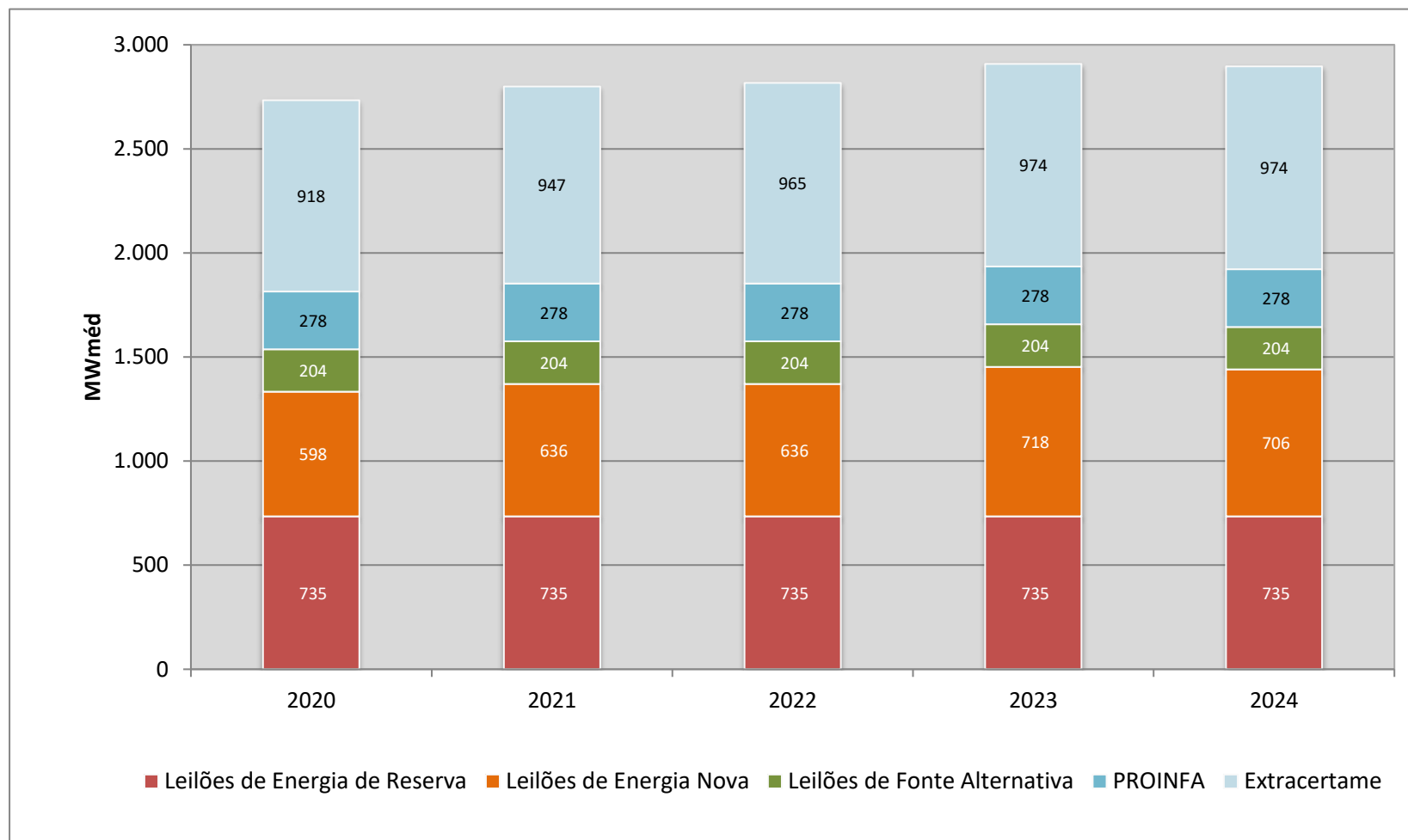
Gráfico 8-6. - Energia contratada e extra certame das usinas vencedoras nos Leilões de Energia
