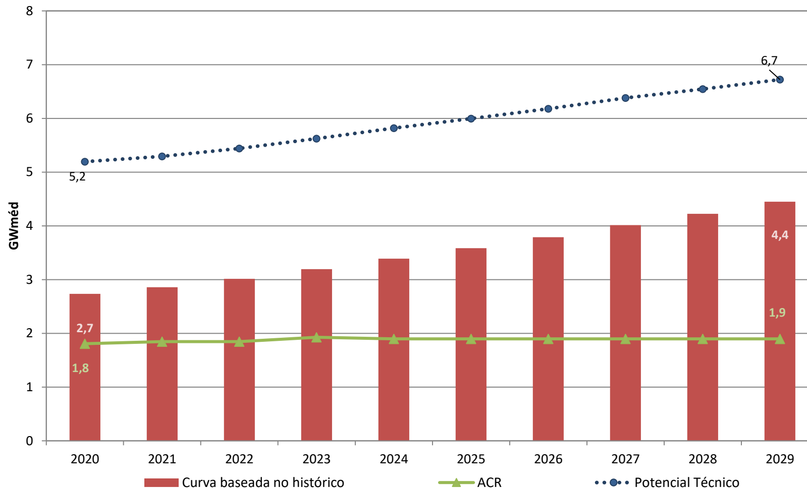
Gráfico 8-7. - Energia contratada no ACR e potencial de exportação de eletricidade gerada por bagaço
