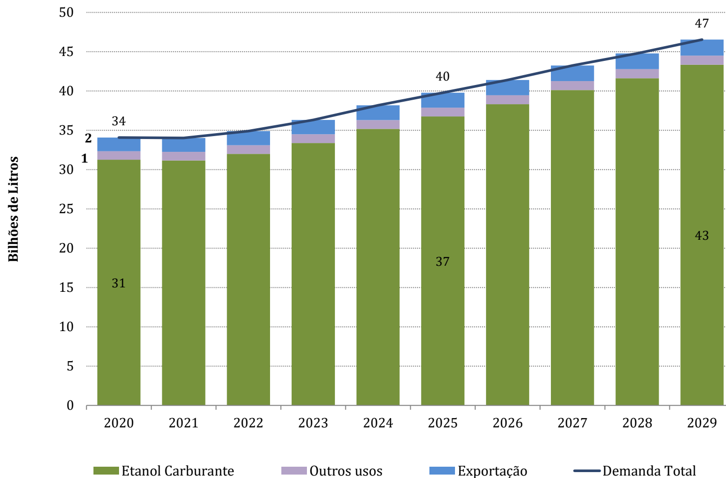
Gráfico 8-5. - Projeção da demanda total de etanol
